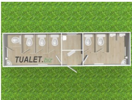
Туалетный модуль Т-440-К с кассой
